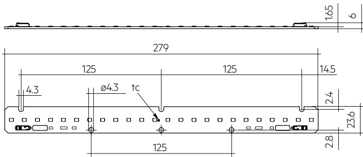
LLE 24x280mm 1250lm HV PRE
